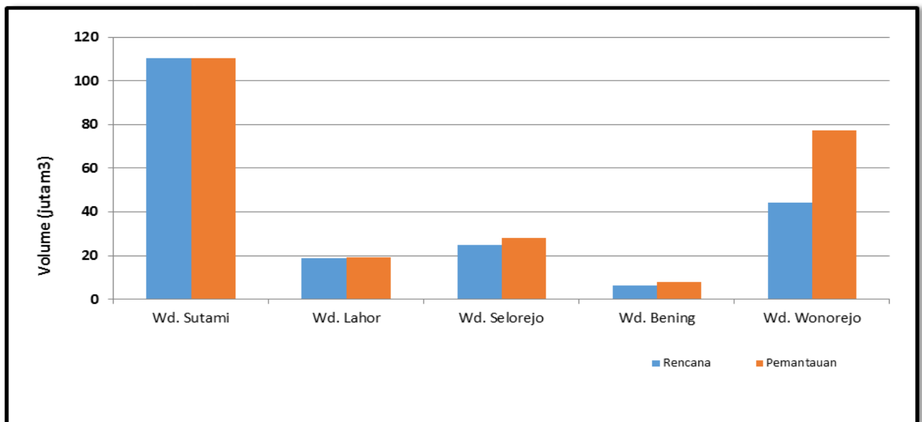
Gambar 4. Perbandingan Volume Rencana dan Pemantauan 5 Waduk Utama di Jawa Timur (Status s/d 31 Agustus 2014)
