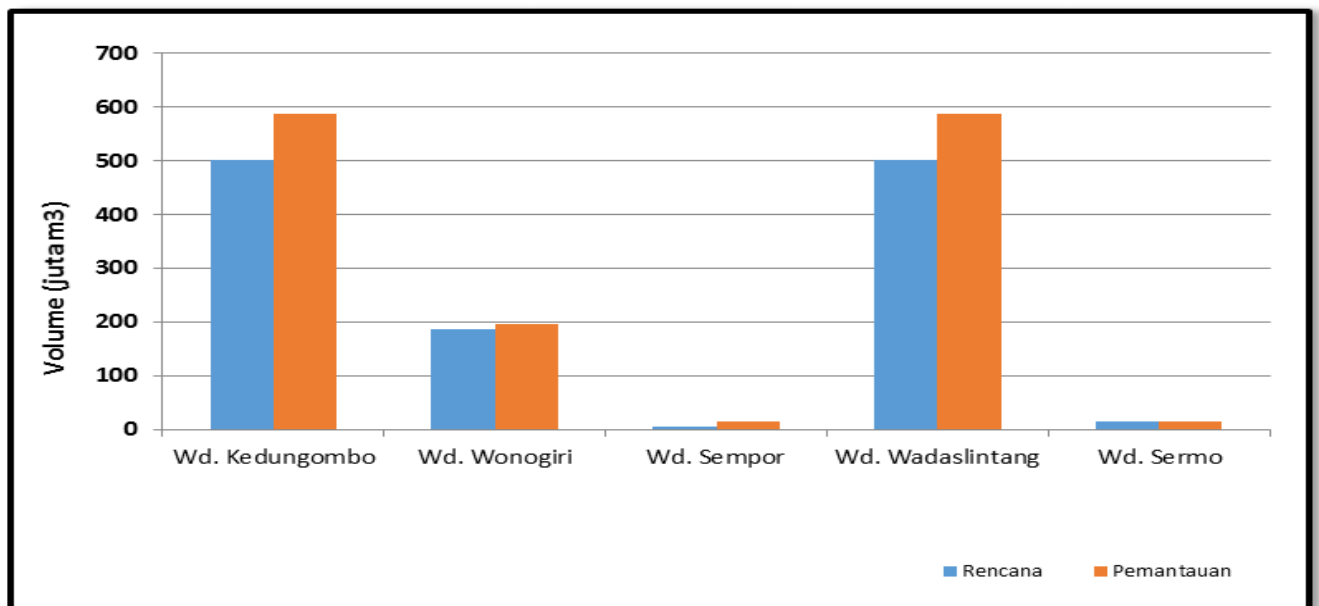
Gambar 3. Perbandingan Volume Rencana dan Pemantauan 5 Waduk Utama di Jawa Tengah dan DIY (Status s/d 31 Agustus 2014)
