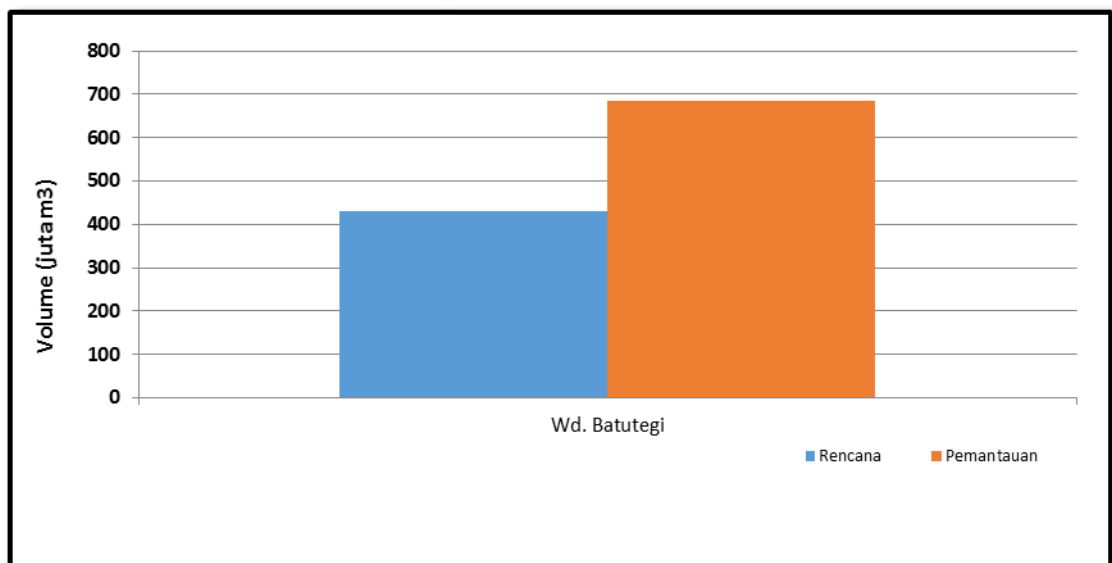
Gambar 7. Perbandingan Volume Rencana dan Pemantauan Waduk Batutegi di Lampung (Status s/d 31 Agustus 2014)
