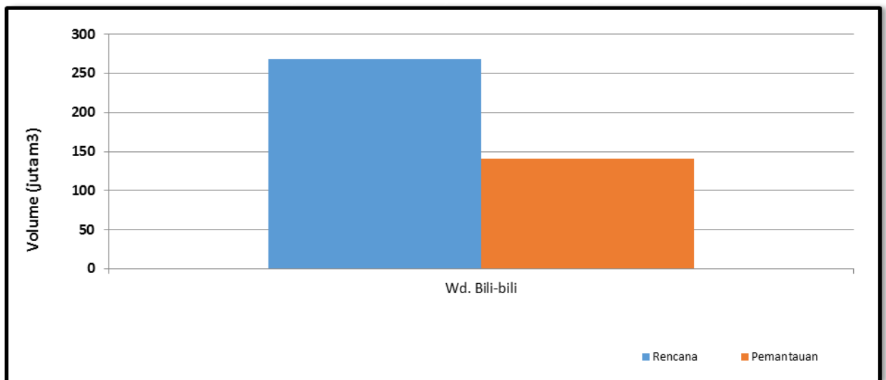
Gambar 5. Perbandingan Volume Rencana dan Pemantauan Waduk Bili-bili di Sulawesi Selatan (Status s/d 31 Agustus 2014)
