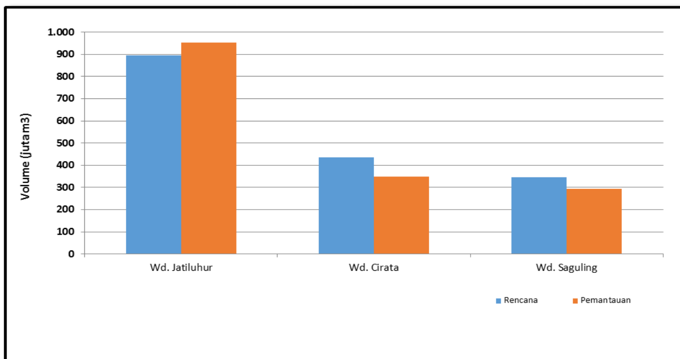
Gambar 2. Perbandingan Volume Rencana dan Pemantauan 3 Waduk Utama di Jawa Barat (Status s/d 31 Agustus 2014)
